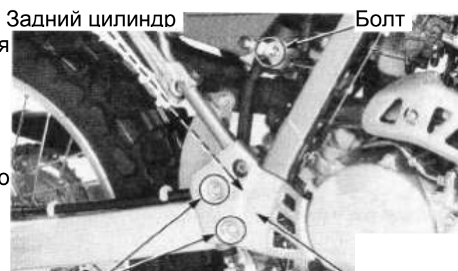
Болты крепления
