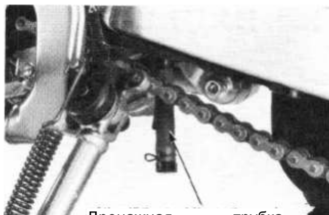
Дренажная трубка камеры сапуна
