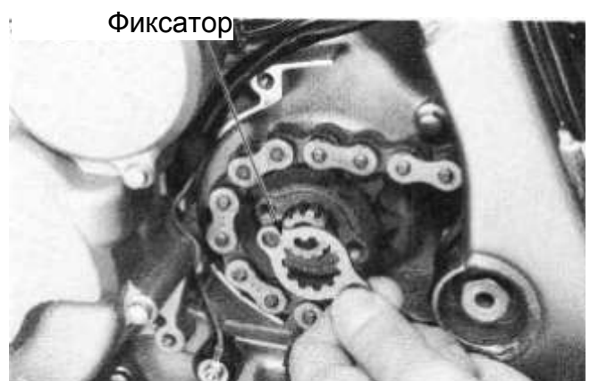
Звёздочка
