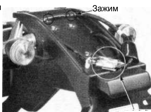
Разъём
