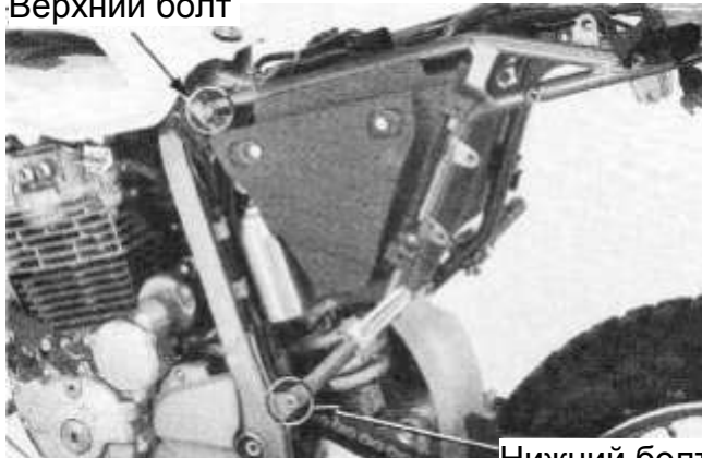
Нижний болт
