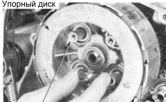
Нажимная пластина
