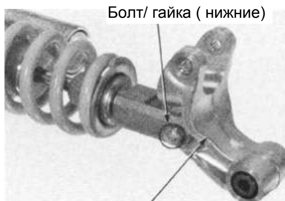
Рычаг амортизатора
