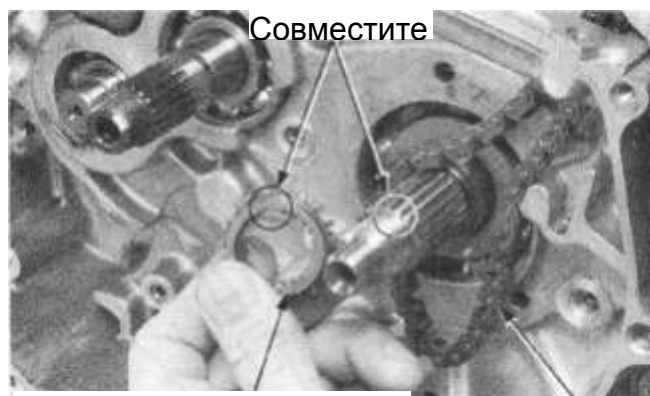
Цепь ГРМ
