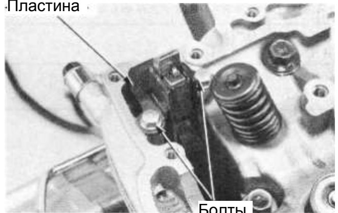
Болты
