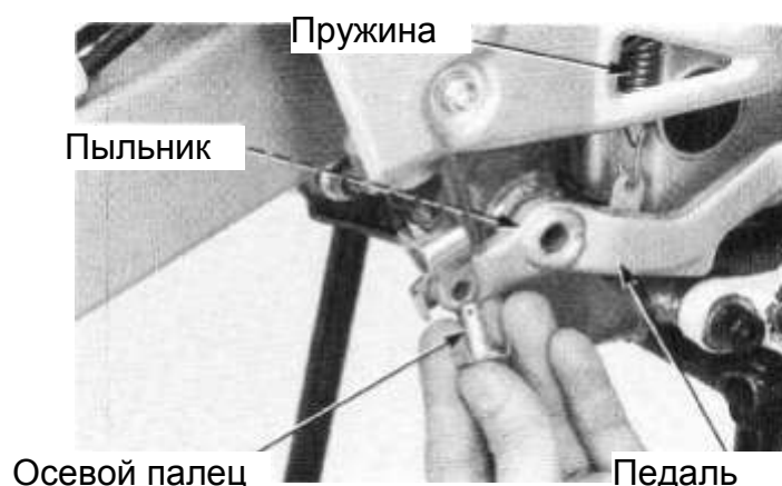
Педаль
