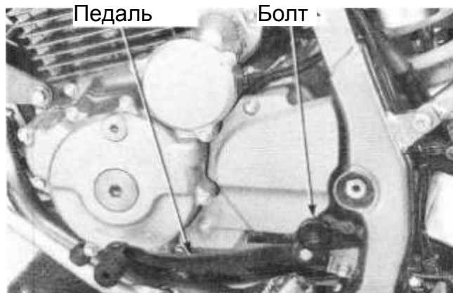
Педаль
