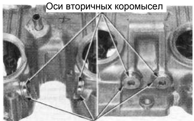
Вторичные коромысла (EX) Вторичные коромысла (IN)
