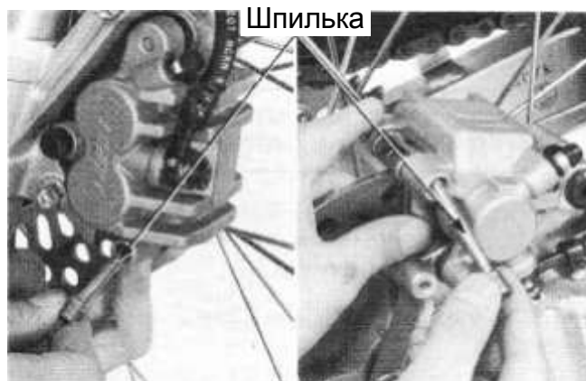
Колодки
