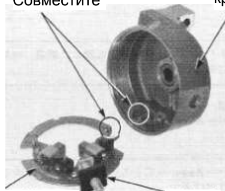
Фиксатор «щётки» в сборе Упор
