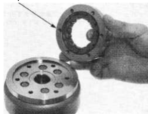
Муфта в сборе
