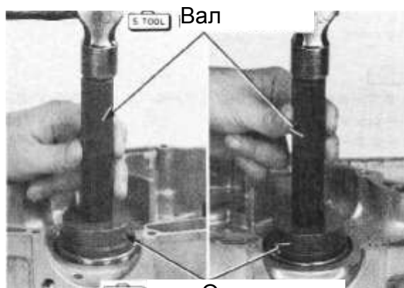
Оправка
