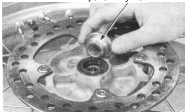
Правая втулка
