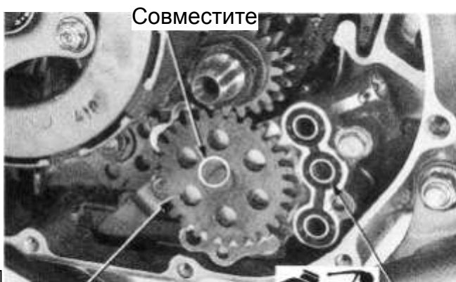
Приводная шестерня
