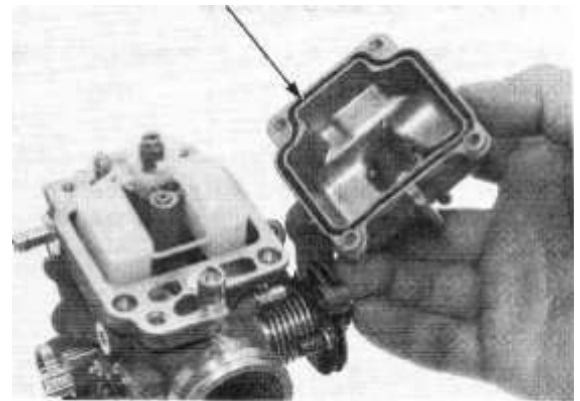
Прокладка
