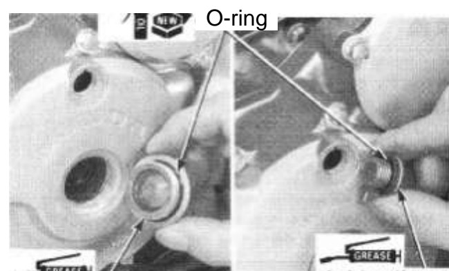
Резьба крышек коленвала и вала ГРМ
