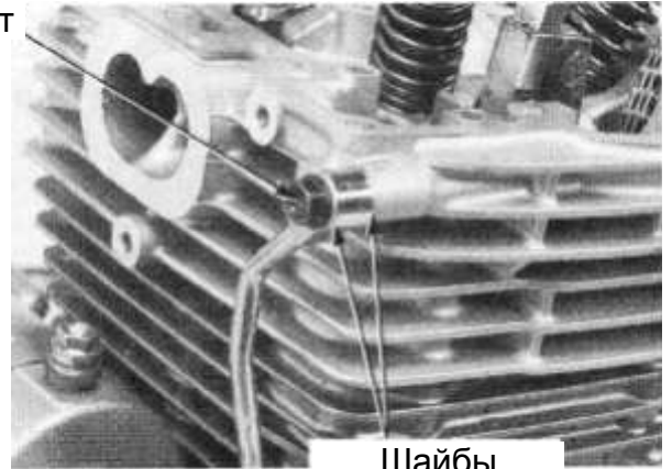
Шайбы
