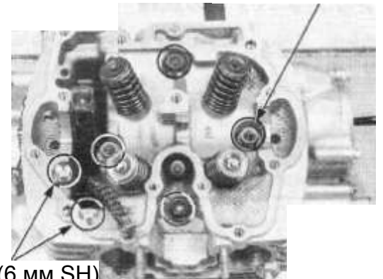
Болты/ шайбы
