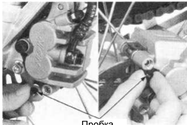
Пробка
