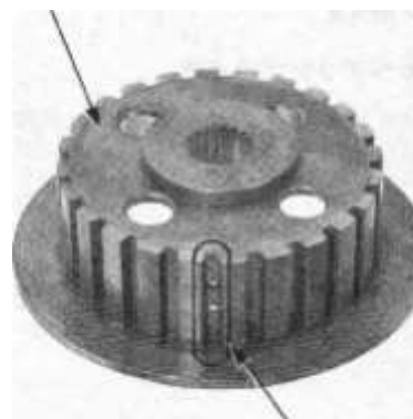
Пазы
