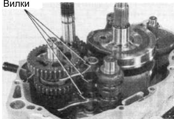
Вилки
