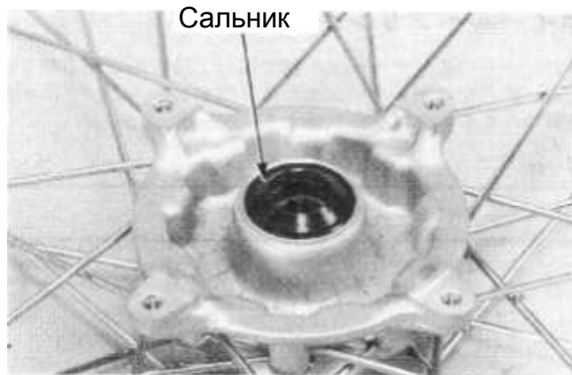
Сальник
