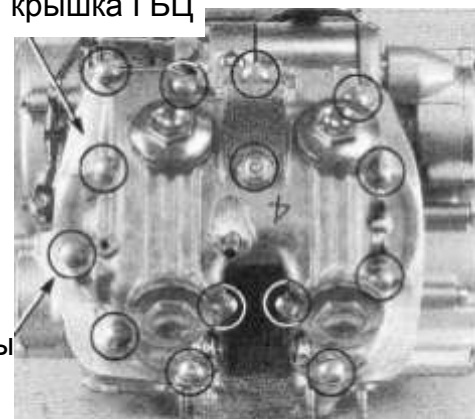
крышка ГБЦ
