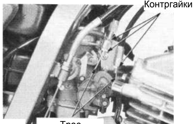
Трос
