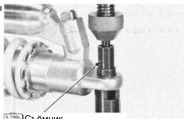
Съёмник
