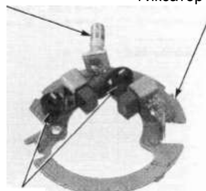
Пружины
