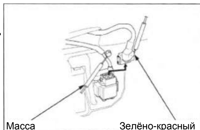
(-) Масса
