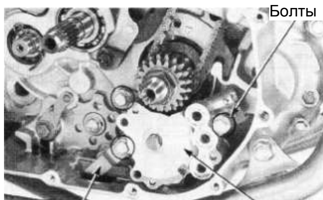
Стопорная пластина
