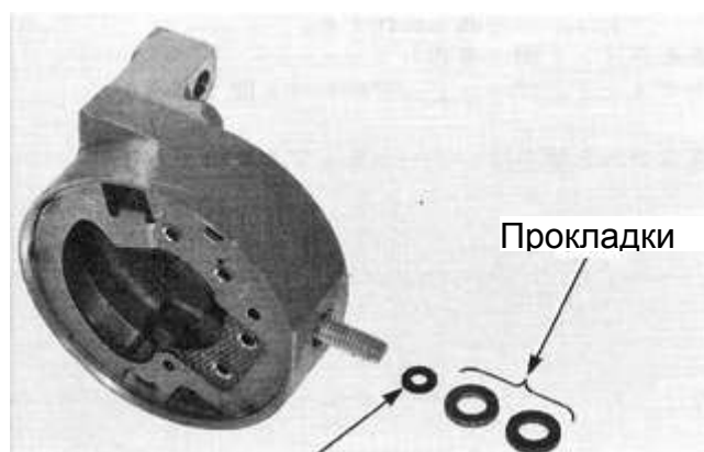
Фиксатор щетки в сборе
