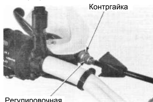
Регулировочная гайка
