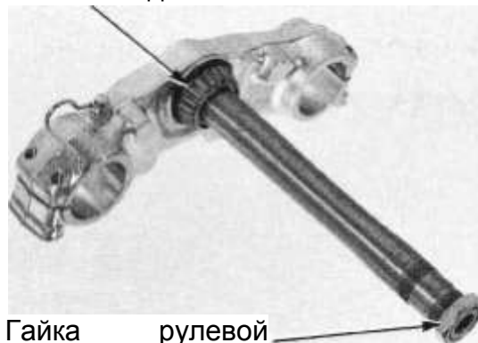
Нижний подшипник / пыльник
