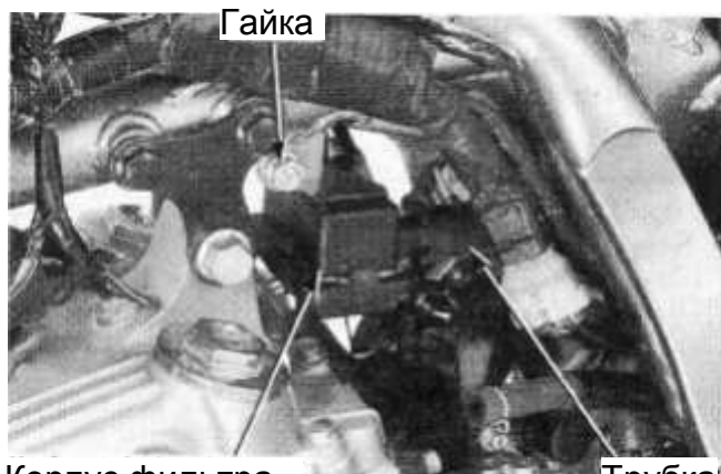
Корпус фильтра
