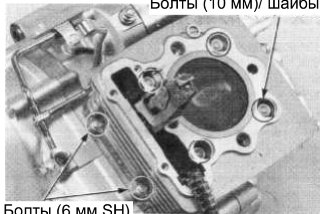
Болты (10 мм)/ шайбы
