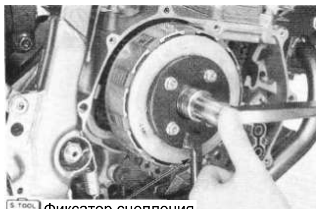
5 TOOL Фиксатор сцепления
